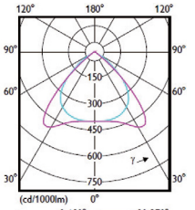
Breitstrahlend (WB)
