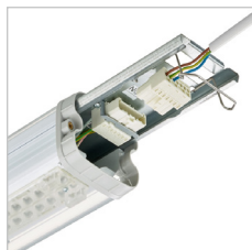
Einfacher und schneller elektrischer Anschluss (WA7)
