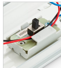
All-in: Der integrierte Lumen-Schalter ermöglicht die einfache Auswahl zweier Leuchtenlichtströme
