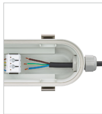
Steckanschlussklemme - Auch zur bauseitigen Durchgangsverdrahtung geeignet.
