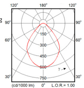
Aluminium Reflektor (UGR19)
