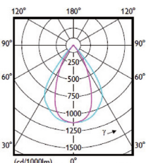
Engstrahlend (NB)
