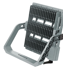
BV Ausführung: Externes Betriebsgerät für entfernte Montage im Karton beigelegt
